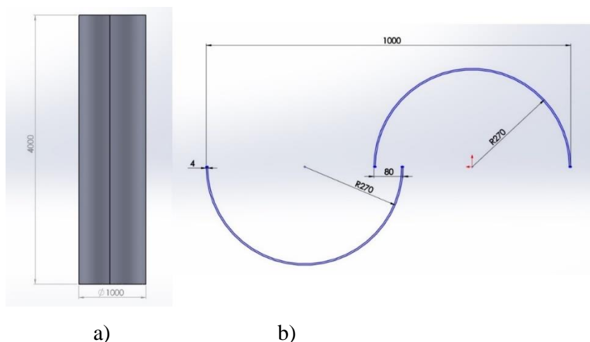
Figura 1. Rotor proposto (unidade em mm): a) Vista frontal; b) Vista superior.
