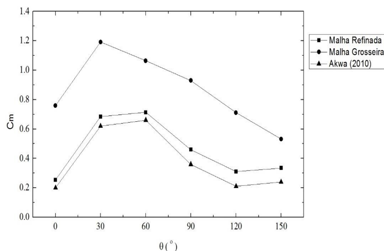
Figura 12. Variação do coeficiente de torque ( C_m ) em relação ao ângulo de incidência de vento obtido com as diferentes malhas estudadas aqui e comparação com os resultados obtidos por Akwa (2010).
