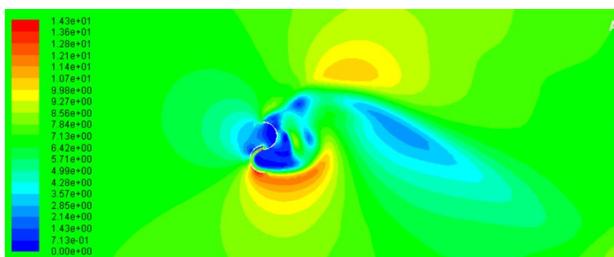
Figura 9. Campo de velocidades no escoamento com o rotor estático, para \theta = 90^\circ e V_o = 7\text{m/s}
