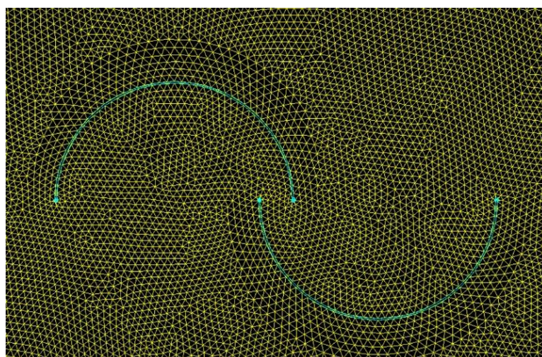
Figura 4. Malha grosseira empregada na região das pás.
