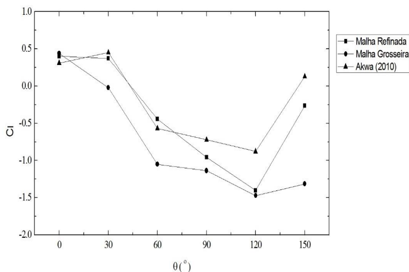
Figura 11. Variação do coeficiente de sustentação ( C_l ) em relação ao ângulo de incidência de vento obtido com as diferentes malhas estudadas aqui e comparação com os resultados obtidos por Akwa (2010).
