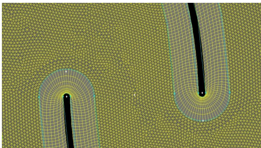
Figura 6. Malha refinada empregada próxima às extremidades das pás.
