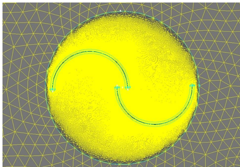
Figura 7. Malha refinada empregada na região de interface.
