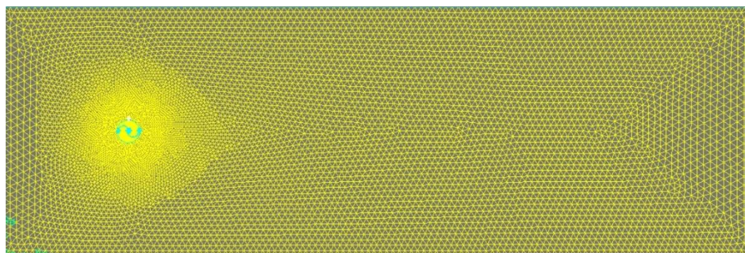
Figura 8. Malha refinada empregada no domínio computacional.
