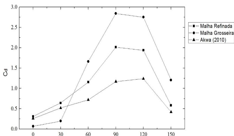
Figura 10. Variação do coeficiente de arrasto ( C_d ) em relação ao ângulo de incidência de vento obtido com as diferentes malhas estudadas aqui e comparação com os resultados obtidos por Akwa (2010).
