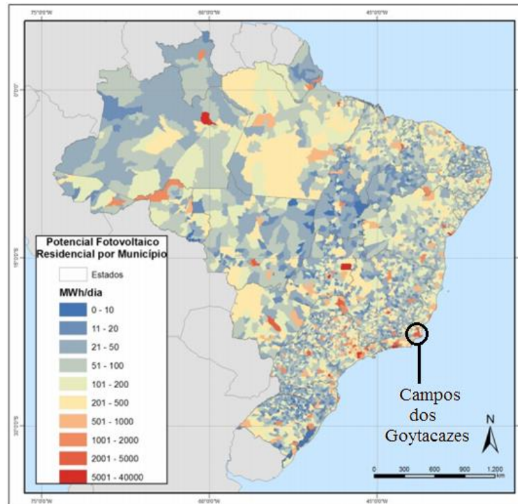
Figura 01. Mapa do Potencial Técnico de Geração Fotovoltaica em Telhados Residenciais por Município. Fonte: EPE (2014).
