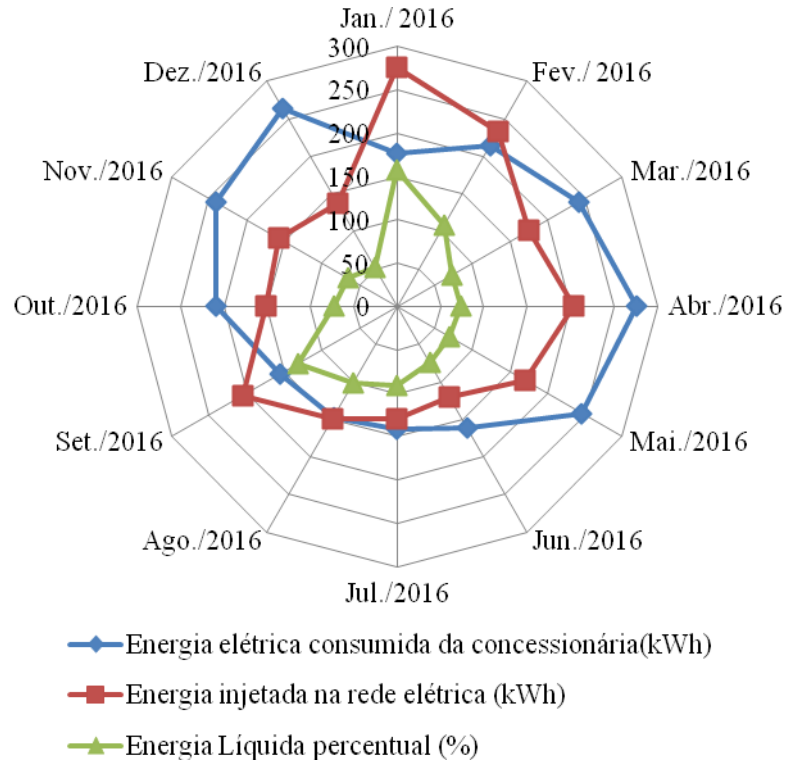
Figura 05. Histórico do consumo mensal de energia elétrica da residência, energia injetada na rede elétrica pelo sistema de ESFV, ambas em kWh, e a energia líquida percentual (%). Fonte: próprios autores a partir dos dados da ENEL.
