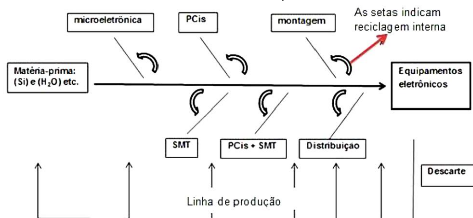
FIGURA 3: DIAGRAMA DE ISHIKAWA DA PRODUÇÃO NO SETOR ELETROELETRÔNICO
