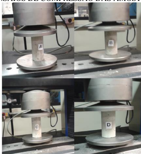
FIGURA 5: ENSAIOS DE COMPRESSÃO DAS AMOSTRAS A, B, C, D.
