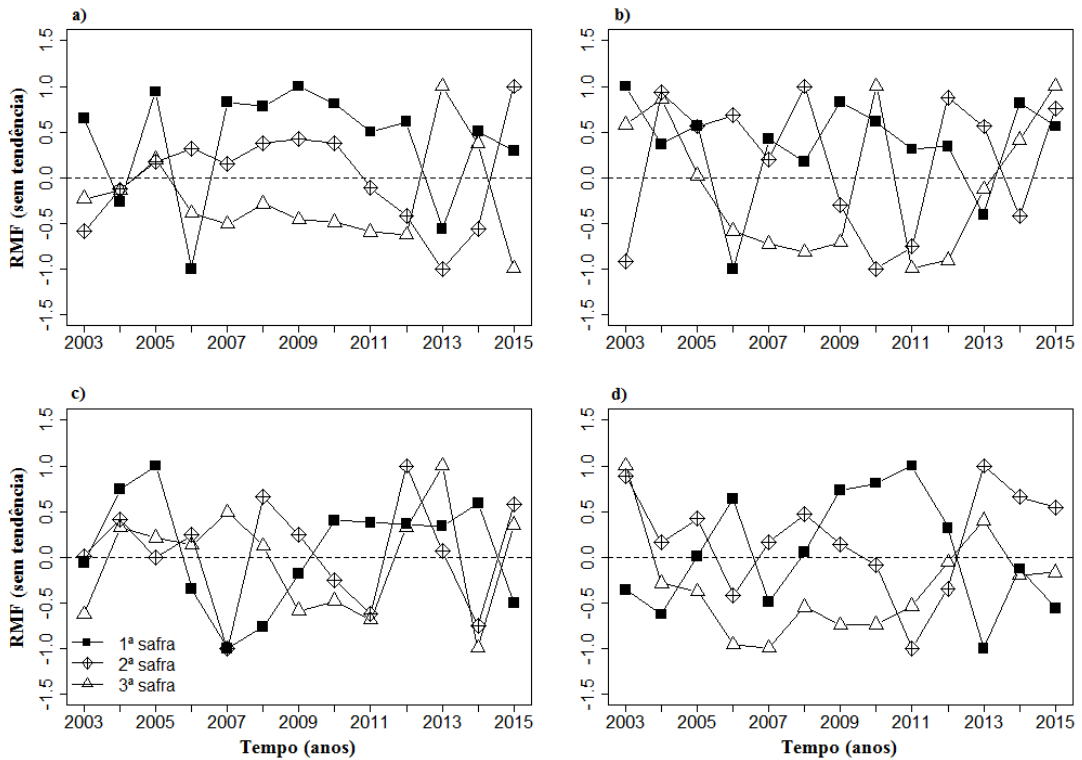
Figura 3 – Série de RMF ( \text{kg.ha}^{-1} ) por safra sem tendência e normalizada para cada macrorregião de MG: a) MMG-1; b) MMG-2; c) MMG-3; d) MMG-4 entre 2003-2015.
