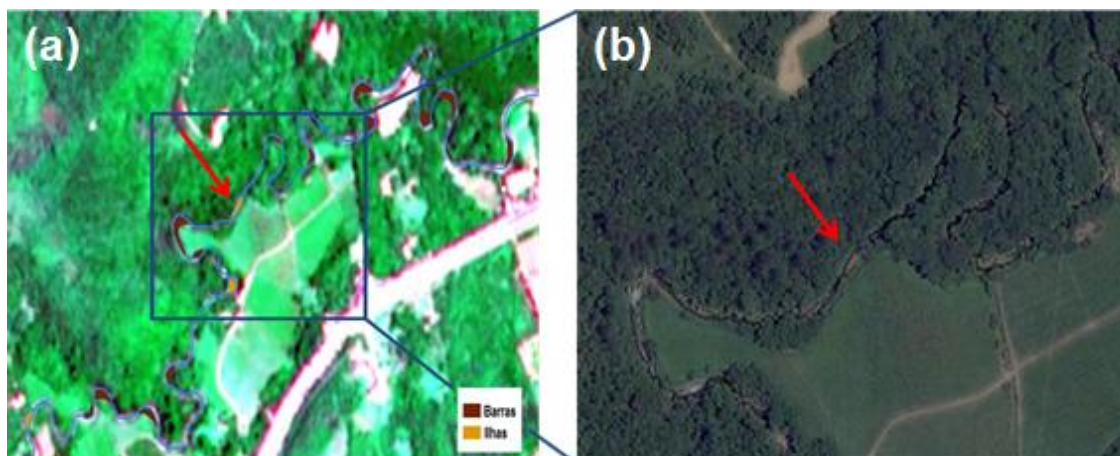
Figura 3 – (a) Identificação das feições fluviais pela imagem SPOT-5 de 2006; (b) confirmação pela imagem do Google Earth
