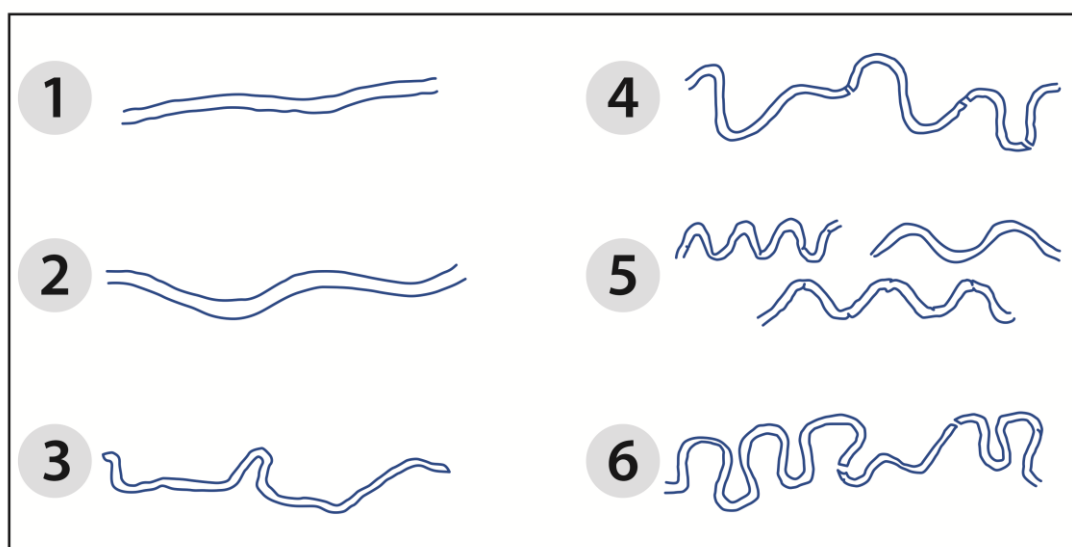
Figura 4 - Classificação de canais fluviais: (1) reto; (2) sinuoso; (3) irregular; (4) meandros irregulares; (5) meandros regulares; (6) meandros tortuosos. Fonte: Kellerhals et al. (1976)
