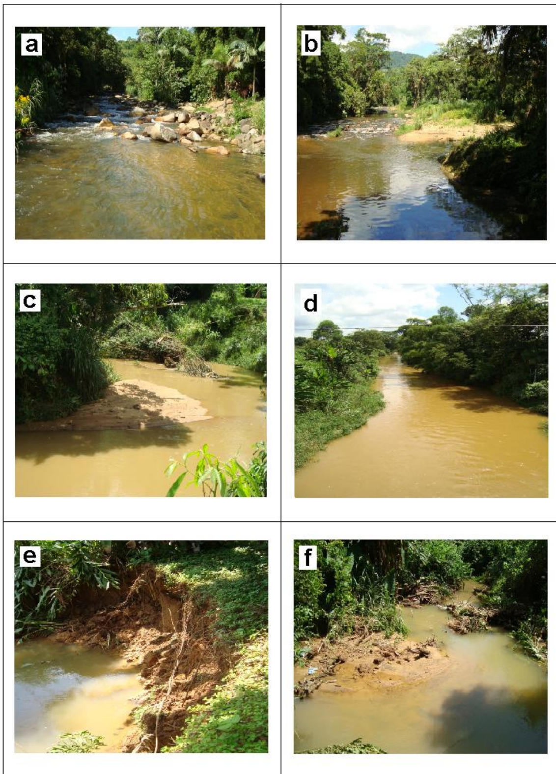
Figura 6 – Características pontuais dos trechos: (a) trecho sem feições fluviais de depósito; (b) barra instável no segmento 4; (c) barra instável no segmento 5; (d) pouca sinuosidade e ausência de deposição no segmento 7 e (e) e (f) afluente instável
