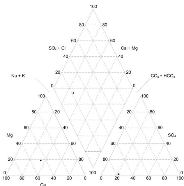
Figura 9 – Diagrama de Piper mostrando a classificação da água coletada na área de estudo em Pontal do Sul.
