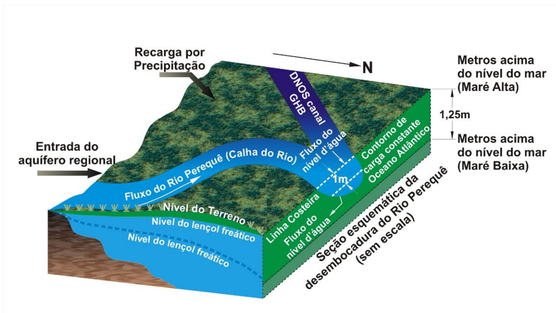
Figura 4 – Modelo Conceitual da zona do aquífero em Pontal do Sul. Fonte: Adaptado de SURESH BABU et al., 2008.
