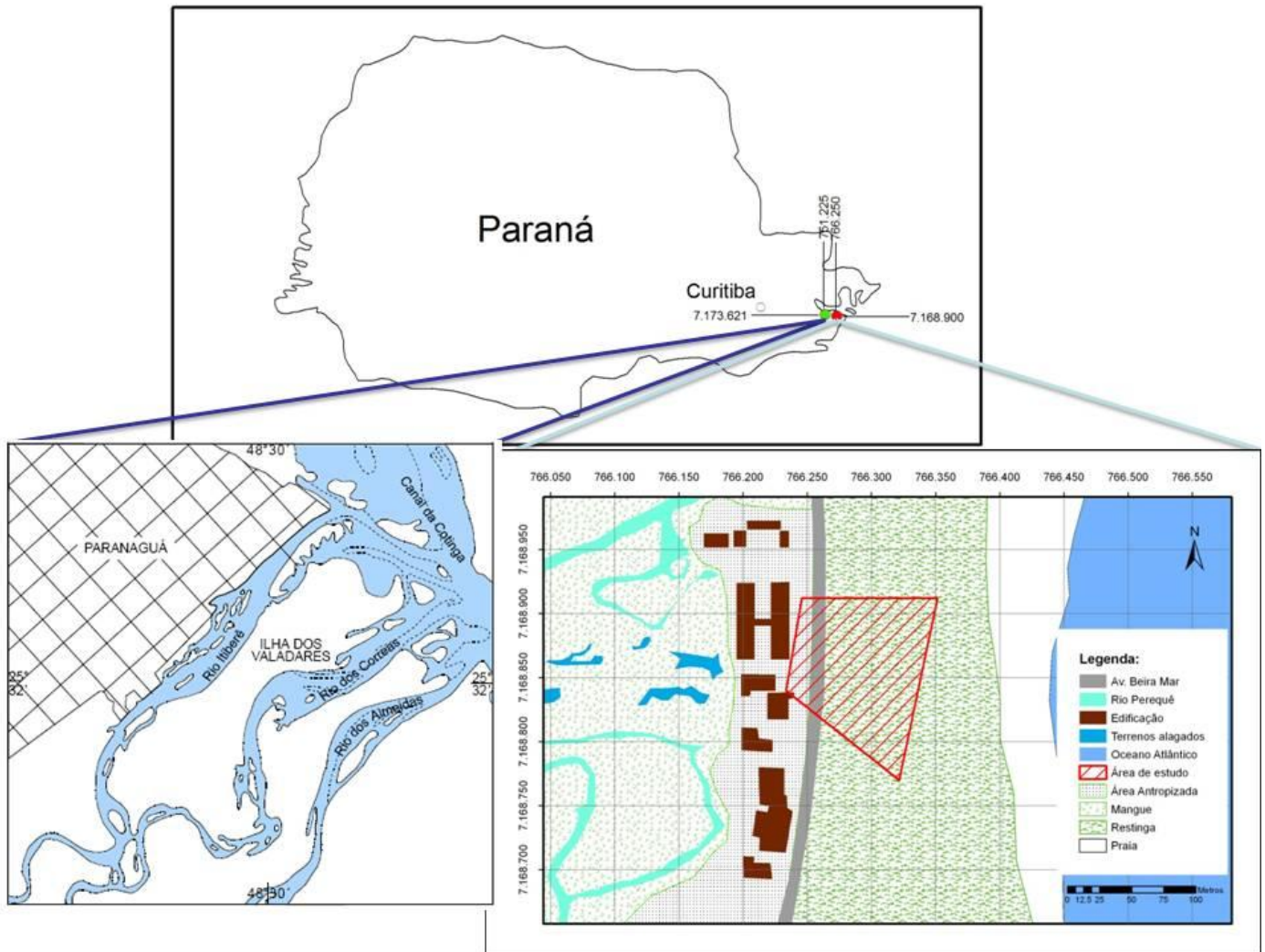
Figura 1 – Localização das áreas estudadas. Para os estudos na Ilha dos Valadares foram utilizados 12 (doze) poços. Em Pontal do Sul foram utilizados 5 (cinco) piezômetros e 3 (três) poços de monitoramento.
