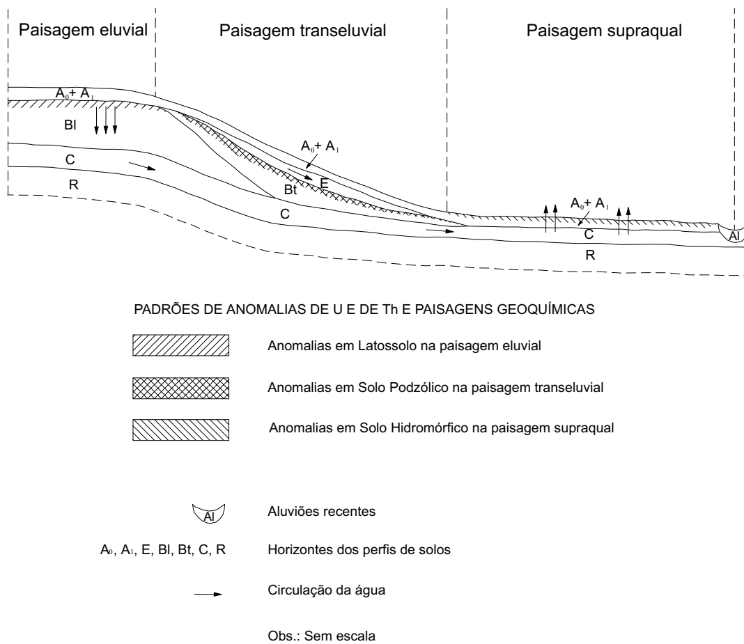
Figura 2: Relações entre sistema de transformação Latossolo-Solo Podzólico, geoformas e padrões de anomalias de U e de Th, em paisagens tropicais úmidas sobre granito (Rebello 2000). Relationships among the Latosol-Podzolic transformation system, geomorphs, and the patterns for U and Th anomalies, in humid tropical landscapes over granite (Rebello 2000).
