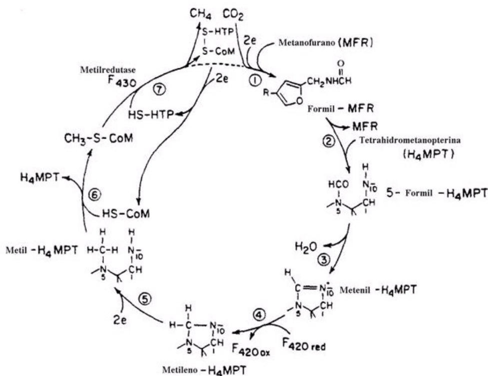
FIGURA 4 – ROTA METABÓLICA DA PRODUÇÃO DE METANO A PARTIR DO CO 2 .
