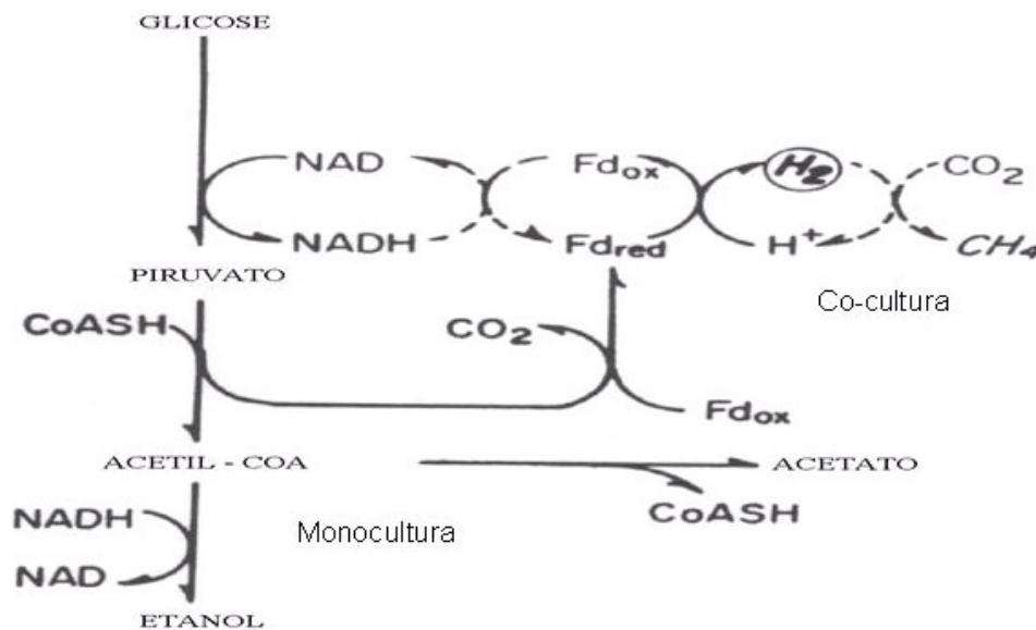
FIGURA 3 – FERMENTAÇÃO DE CARBOIDRATOS POR Ruminococos albus .
