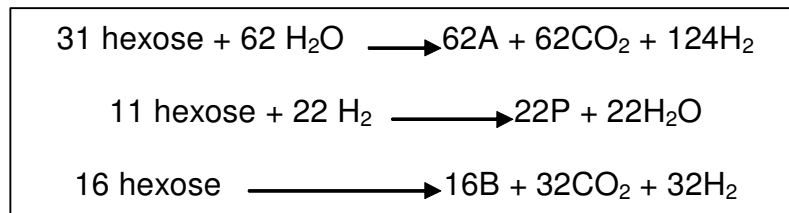
FIGURA 2 – ESQUEMA DE PRODUÇÃO DE AGV NO RÚMEN.
