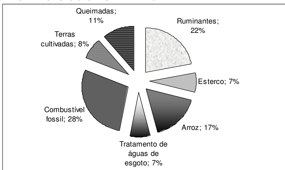
FIGURA 1 – FONTES ANTRÓPICAS GLOBAIS DE METANO.
