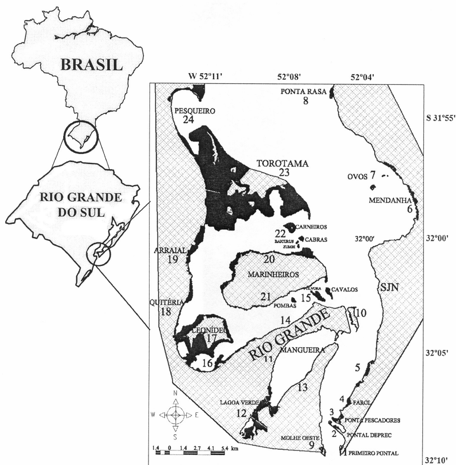
FIGURA 1 – ESTUÁRIO DA LAGOA DOS PATOS (RS, BRASIL) COM A LOCALIZAÇÃO DAS 24 UNIDADES DE MARISMAS (ÁREAS ESCURAS) NOS MUNICÍPIOS DE RIO GRANDE (RG) E SÃO JOSÉ DO NORTE (SJM).
