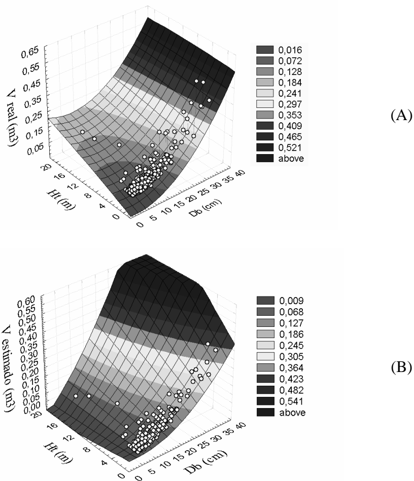
Figura 3. Relação das variáveis de volume ( m^3 ) real (A – equação de Smalian) e estimado (B – equação ajustada) com a altura total (Ht) e o diâmetro da base (Db) de árvores de cerrado em Planaltina de Goiás.
