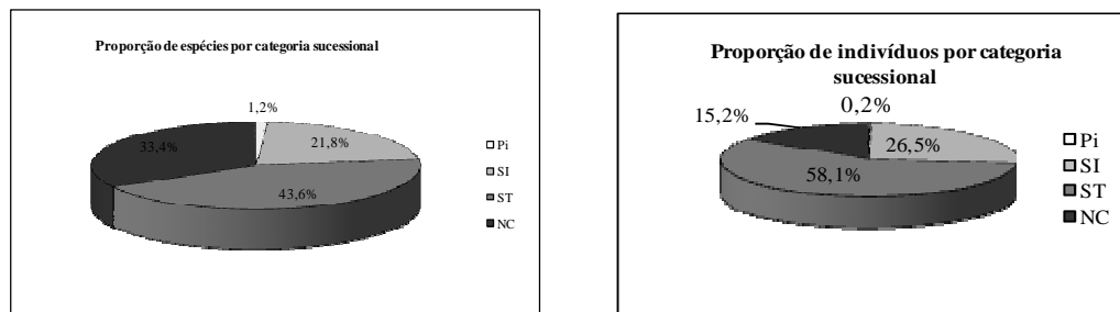
Figura 2. Categorias sucessionais, representadas em porcentagem das espécies e indivíduos amostrados no fragmento da Reserva Particular do Patrimônio Natural Cafundó.
