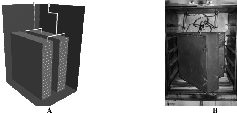
Figura 1. Projeto das caixas para instalação no interior da estufa, visando injeção de nitrogênio gasoso: A) Tubulação à direita para entrada do gás, tubulação à esquerda para a saída do gás; B) Visão geral do sistema instalado na estufa.
