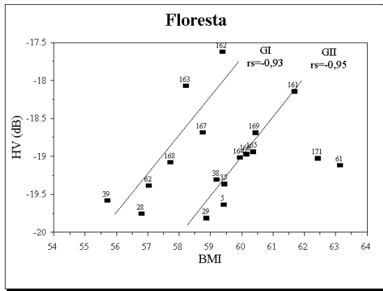
Figura 2 –Diagrama de dispersão do \sigma^\circ da polarização HV com o índice BMI para a classe Floresta. O índice BMI é expresso em escala linear para permitir o uso direto de algoritmos de processamento de imagem.
