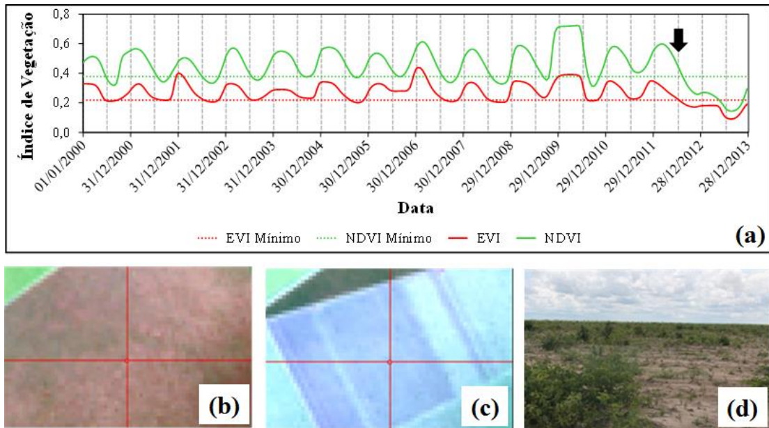
Figura 6: Séries temporais de EVI e de NDVI de um ponto em Luís Eduardo Magalhães (latitude: 11 ° 59' 27,50" S; longitude: 45 ° 58' 48,16" W) com correspondentes limiares de desmatamento de uma formação savânica (a). Em meados de 2012, as séries temporais cruzam os limiares de desmatamento (seta preta). O desmatamento nesse período pode ser confirmado pelos recortes de cenas do satélite Landsat de 3 de setembro de 2011 (b) e 8 de setembro de 2013 (c). Fotografia de campo obtida em fevereiro de 2014 (d) também indica que a área foi desmatada. Foto: R. Trevizam.
