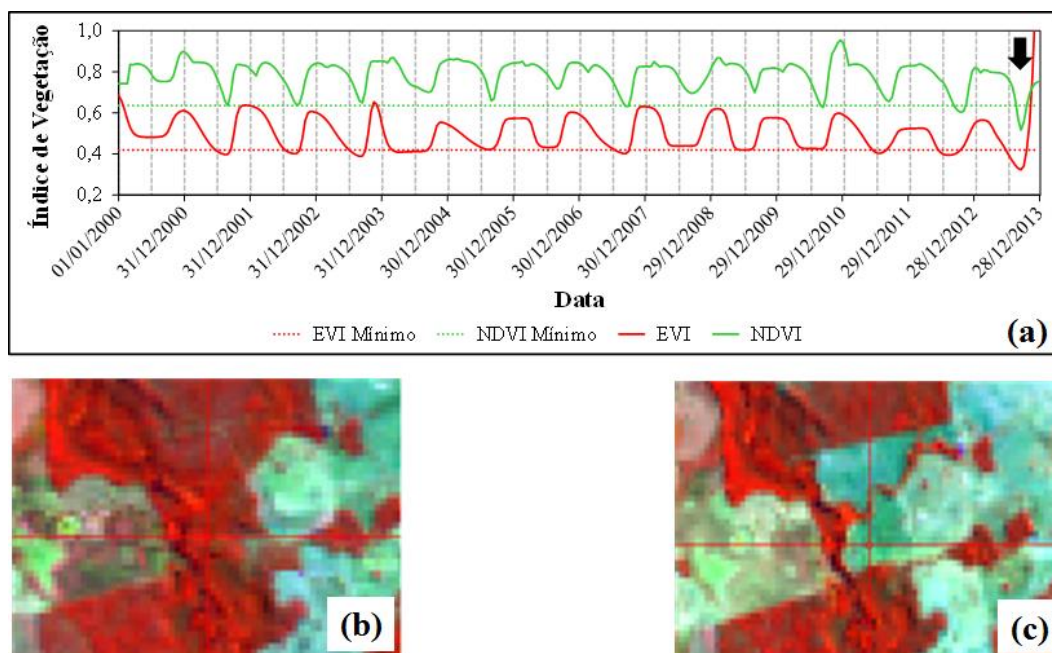
Figura 5: Séries temporais de EVI e de NDVI de um ponto em SMA (latitude: 13^{\circ} 20' 42,46'' S; longitude: 49^{\circ} 58' 52,29'' W) com correspondentes limiaries de desmatamento de uma formação florestal (a). Em meados de 2013, as séries temporais cruzam os limiaries de desmatamento (seta preta). O desmatamento nesse período pode ser confirmado pelos recortes de cenas do satélite Landsat de 1 de agosto de 2012 (não desmatado) (b) e 12 agosto de 2013 (desmatado) (c).
