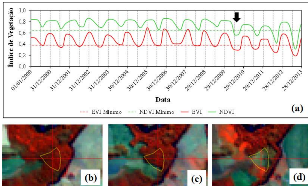
Figura 4: Séries temporais de EVI e de NDVI de um ponto em Jataí (latitude: 17^{\circ} 58' 54,79'' S; longitude: 51^{\circ} 41' 37,54'' W) com correspondentes limiaries de desmatamento de uma formação florestal (a). Em meados de 2010, as séries temporais cruzam os limiaries de desmatamento (seta preta). O desmatamento nesse período pode ser confirmado pelos recortes de cenas do satélite Landsat de 1 de agosto de 2009 (não desmatado) (b), 3 de julho de 2010 (desmatamento nas adjacências do polígono) (c) e 22 de julho de 2011 (desmatado) (d).
