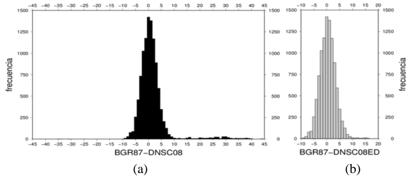
Figura 9: Histograma de las diferencias BGR87-SyS16.1 cruda (a), izquierda y editada (b), derecha.
