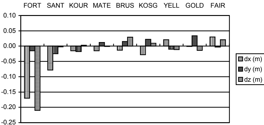
FIGURA 2 – DIFERENÇAS ENTRE COORDENADAS CALCULADAS E DIVULGADAS – ITRF93
