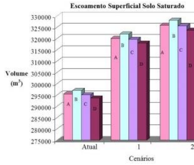
Figura 10. Volumes de escoamento superficial gerados para a sub-bacia Restante. Figure 10. Runoff volumes generated for sub-basin Restante.
