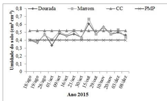
Figura 6. Monitoramento da umidade de um Cambissolo Húmico Háplico sob cultivo de duas variedades de linho (marrom e dourado) ao longo do ciclo da cultura no ano de 2015.
