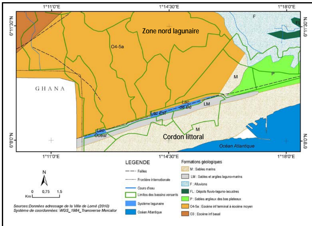
Figure 1 : Ensemble géologique et hydrographique de la zone d'étude
