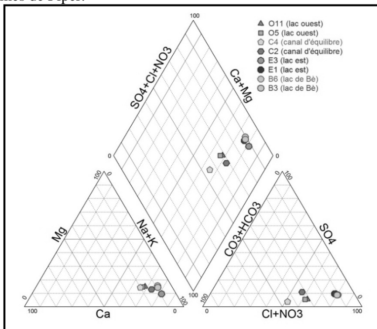
Figure 5 : Diagramme de Piper des eaux
