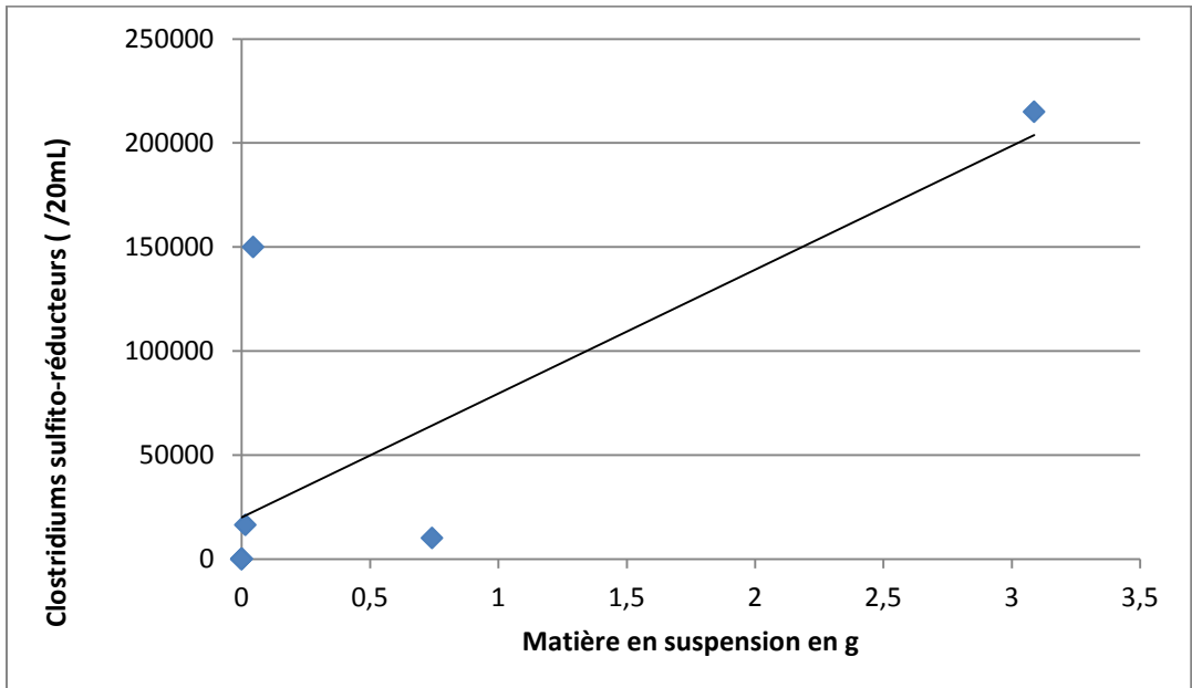
Figure 11 : Evolution du nombre de colonies de clostridium sulfito-réducteurs en fonction de la MES.
