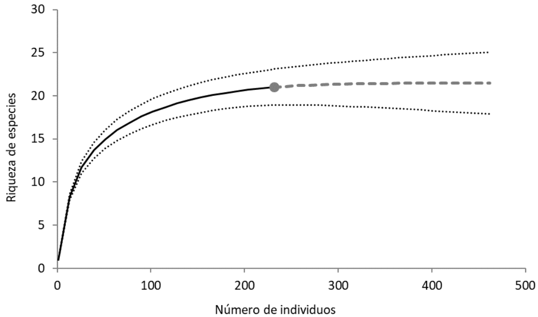
Figura 2. Curva de rarefacción entre la riqueza de especies y el número de individuos para las plantaciones del higo Ficus carica , en el sector norte del Cinturón Verde de la ciudad de Santa Fe, provincia de Santa Fe, Argentina. La línea sólida muestra la interpolación y la línea cortada la extrapolación, con base en el número de individuos. \pm intervalos de confianza del 95% están representados por las líneas punteadas.
