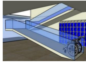
Gambar 16 Solusi desain ramp menuju lt.2. (digambar : Tim Peneliti, 2018)
