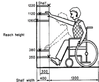
Gambar 8. Ukuran tinggi lemari buku yang mudah dijangkau orang disabilitas (250 – 1220 mm). (Sumber : Human dimension (Panero and Zelnik)
