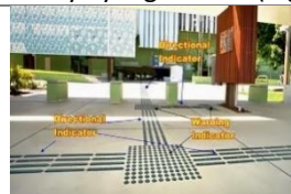
Gambar 24 Solusi desain sirkulasi jalan dengan guiding block. (digambar : Penulis, 2018)
