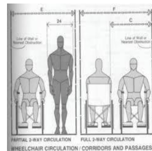
Gambar 9. Ergonomis dan jalur sirkulasi bagi disabilitas. Sumber : Human dimension (Panero and Zelnik)
