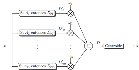
Figura 2 Salida del motor de inferencia tipo SAM Fuente: elaboración de los autores
