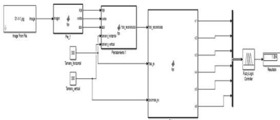
Figura 11. Diagrama de bloques de simulación de Simulink® de Matlab Vr2015a®
