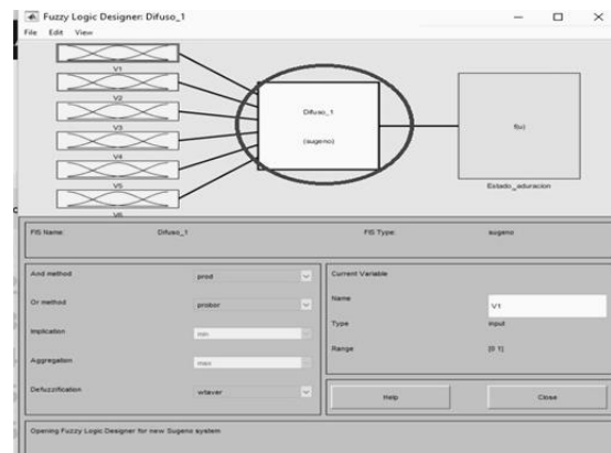
Figura 10. Fuzzy Logic Designer de Matlab Vr2015a con las entradas definidas de la caracterización de las fotos del Arazá
