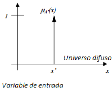
Figura 1. Forma de la entrada Singleton Fuente: elaboración de los autores
