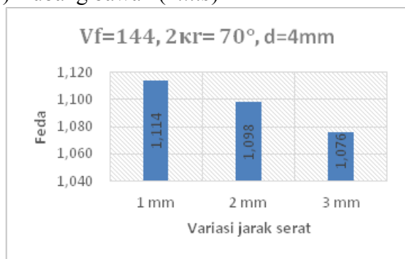
Gambar III Grafik perbedaan Feda pada setiap variasi jarak yang ditentukan pada lubang sisi atas dan bawah.
