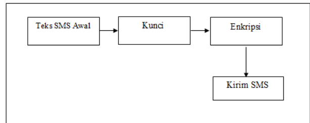
Gambar 1. Proses Enkripsi
