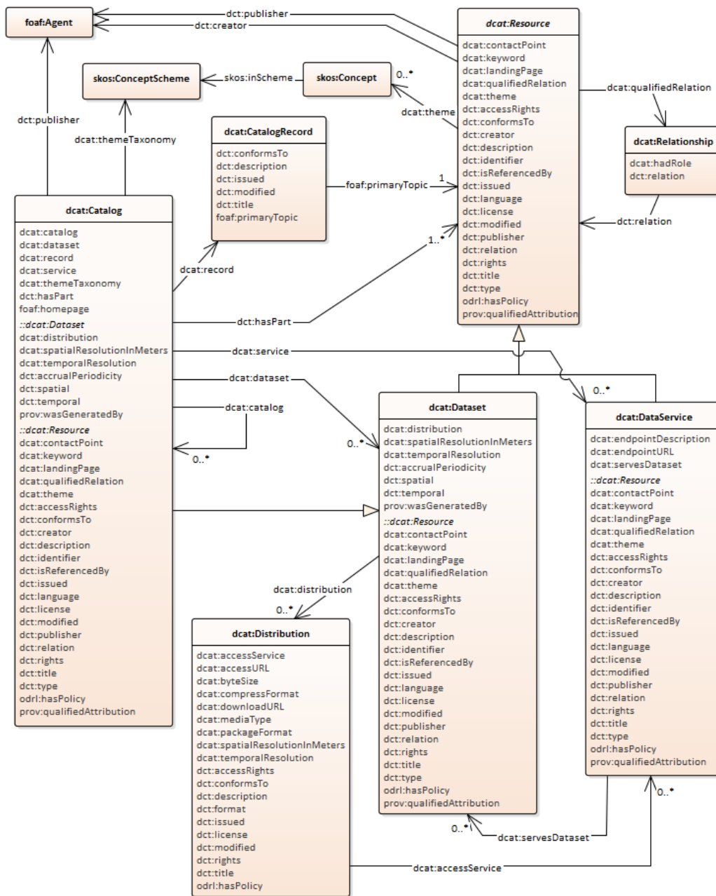
Figura 3. Rappresentazione grafica del modello DCAT (W3C 2020)
