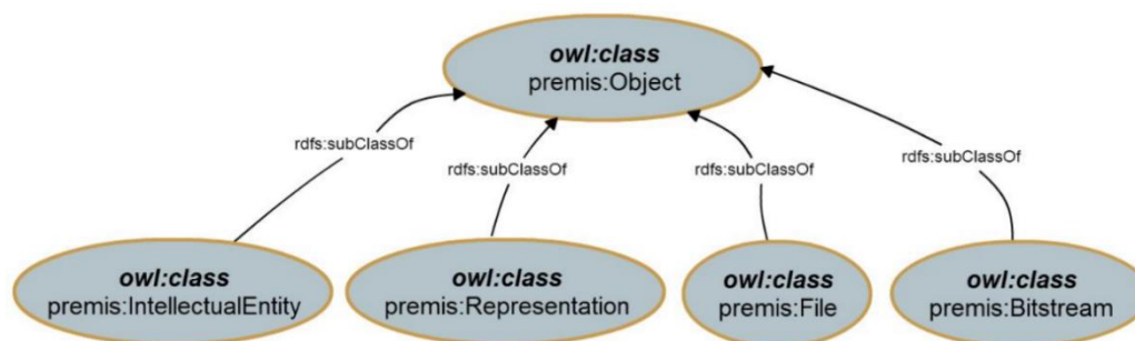
Figura 4. I quattro tipi di oggetto dell'ontologia PREMIS
