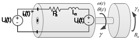
รูปที่ 1 วงจรสมมูลของมอเตอร์ไฟฟ้ากระแสตรง
