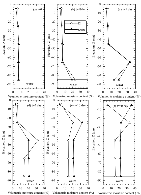
รูปที่ 9 เปรียบเทียบความสัมพันธ์ระหว่างความลึกและความชื้นดิน และระหว่างน้ำใต้ดินจืดและน้ำใต้ดินเค็มสำหรับแห้งดินที่เป็นดินร่วนปนทรายที่ (a) ที่เวลาเริ่มต้น (b) 10 ชั่วโมง (c) 1 วัน (d) 5 วัน (e) 10 วัน (f) 20 วัน
