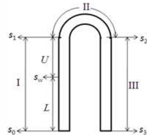
Gambar 1. Sistem koordinat-s pada siphon (Nurhayati dkk., 2015).
