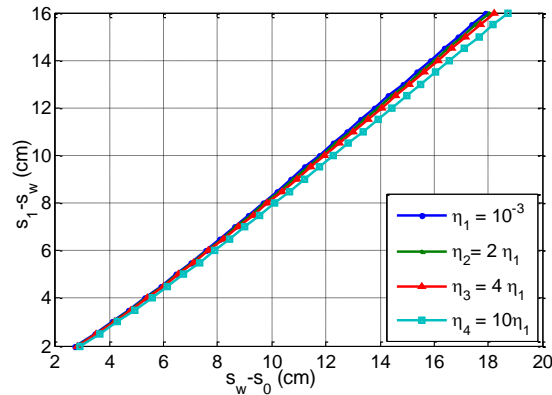
Gambar 3. Grafik terjadinya aliran pada batas segmen II and III untuk \rho 1000 kg/m 3 , diameter dalam pipa 6 mm, dan variasi nilai \eta yaitu 10^{-3} N. s/m 2 (—), 2 \times 10^{-3} N. s/m 2 (—), 4 \times 10^{-3} N. s/m 2 (—), dan 10^{-2} N. s/m 2 (—).
