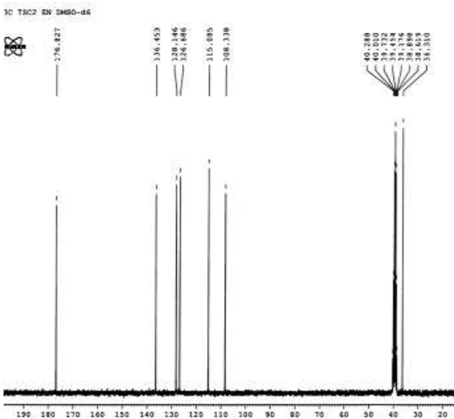
Figura 10 Espectro de RMN- ^{13}\text{C} para el compuesto \text{TSC}^2
