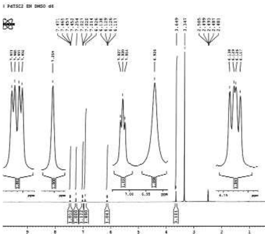
Figura 11 Espectro de RMN- 1 H del complejo de paladio(II), Pd(TSC 2 ) 2
