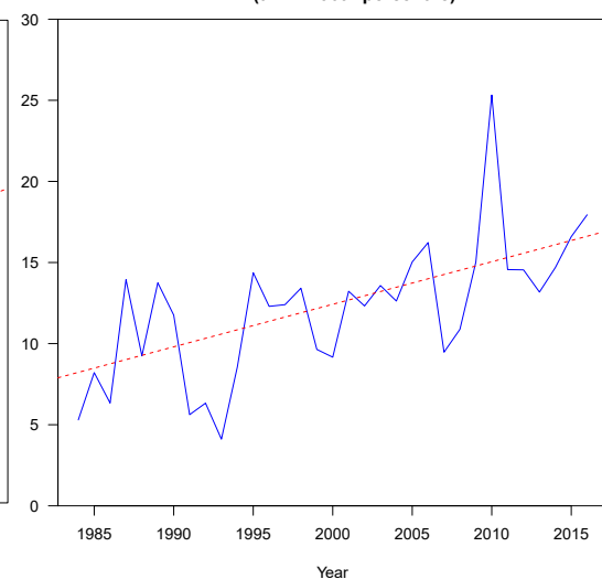
b) Warm nights (Wnights, %)
