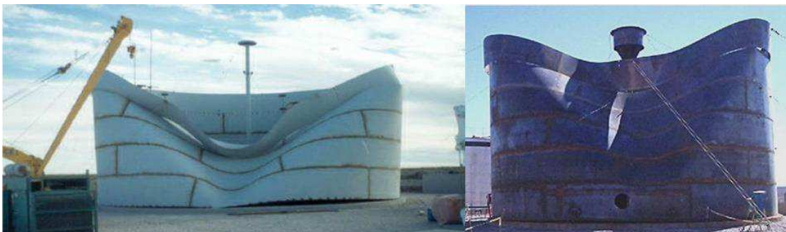
(a) (b) Figura 1: Tanques de petróleo en construcción en el norte de la Patagonia, que colapsaron a velocidades del viento muy inferior a las de diseño.
