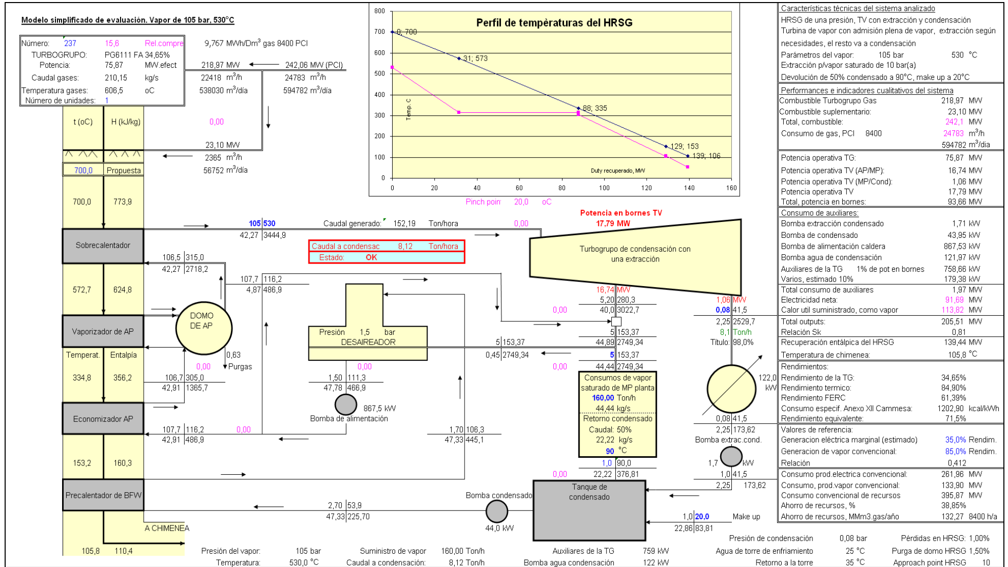
Figura 5: Diagrama de un sistema de cogeneración con ciclo combinado (CC, CHP) con turbina de vapor de condensación con una extracción operando con combustión suplementaria
