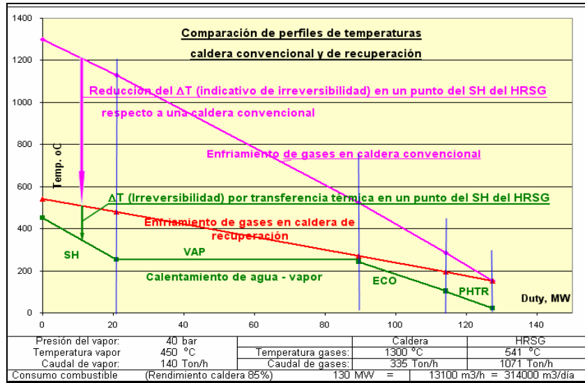
Figura 3: Comparación de los perfiles de temperaturas de una caldera convencional y de recuperación.
