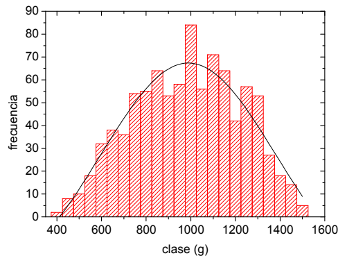
Figura 1: Histograma del ensayo de tracción correspondiente al proceso de soldadura.
