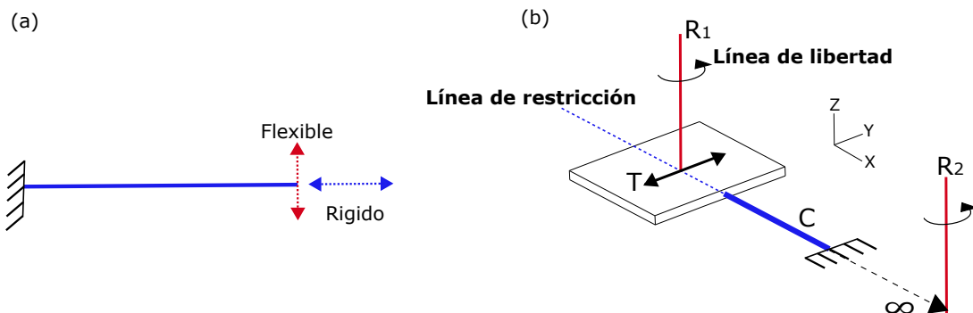
Figura 2: (a) Viga esbelta, equivalente a una restricción ideal; (b) Movimiento plano de un cuerpo con una restricción de viga.
