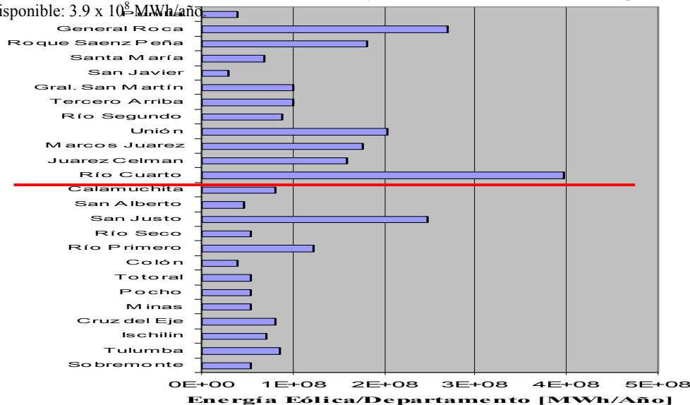
Figura 2: Energía eólica anual por departamento de la provincia de Córdoba.
