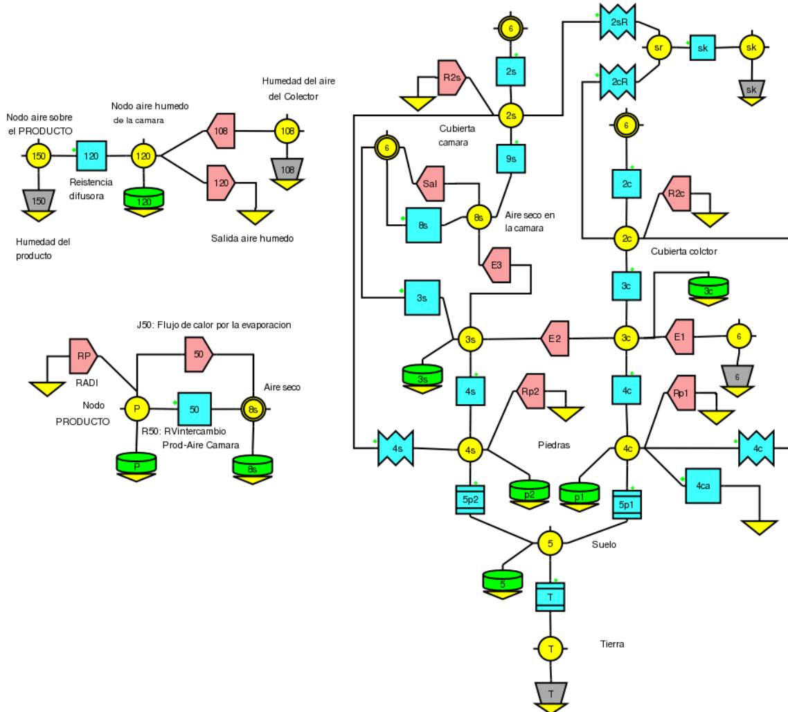
Fig. 4. Diagramas higrotérmicos Simusol del secadero
