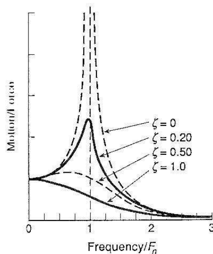
Figura 5: Amplificación dinámica en función de la frecuencia y del amortiguamiento
