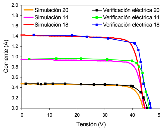
Figura 8. Ensayo eléctrico funcional y simulación de los módulos 20 (1 cadena), 14 (2 cadenas) y 18 (3 cadenas) del EQM.
