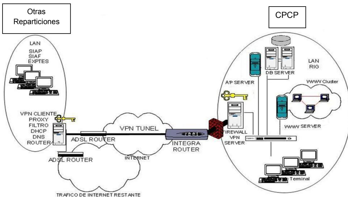
Figura 3. Arquitectura Existente
