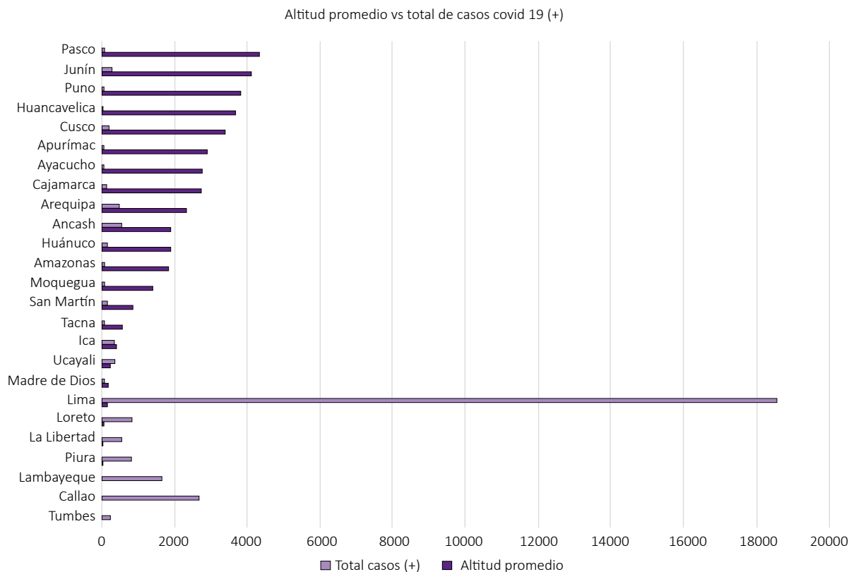
Figura 1. Altitud promedio en relación a casos confirmados COVID 19. Las zonas con una altitud promedio por encima de los 2700 msnm presentan un menor número de infectados COVID 19 (De Pasco a Cajamarca) a diferencia de las zonas con una altitud promedio de 0-600 msnm (De Tacna a Tumbes).
