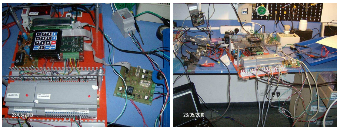
Figura 8 (izq) Armado final del equipo SISMED/C + Placa Interfase Desele (der) Calibración del SISMED/C – 23/5/2010
