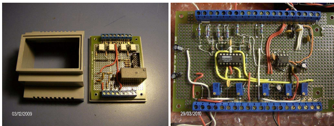
Figura 6 (izq) – Interfase lógica Diesel/Inverter (instalada y en funcionamiento desde 12/09) y (der) Entrada de Canales Analógicos (ambas placas basadas en proto-boards desarrollados por L&R Ingeniería)
