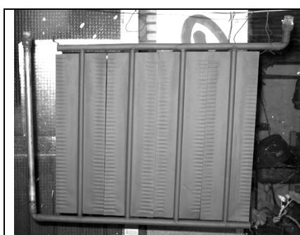
Figura 4: placa captadora terminada
