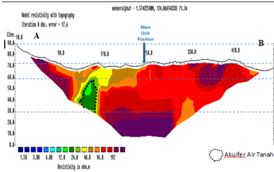
Gambar 2. Cross section bawah permukaan tanah Lintasan 1
