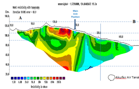
Gambar 5. Cross section bawah permukaan tanah Lintasan 4
