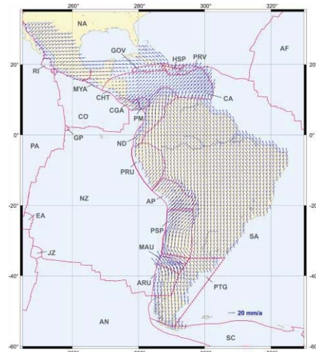
Fig. 4. Campo de velocidades VEMOS2015 [11].
