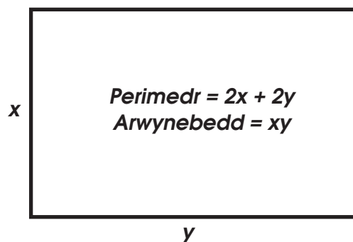
Ffigur 1: Pa gymhareb o x ac y sy'n rhoi'r arwynebedd mwyaf ar gyfer petryal gyda pherimedr penodol, P ?
