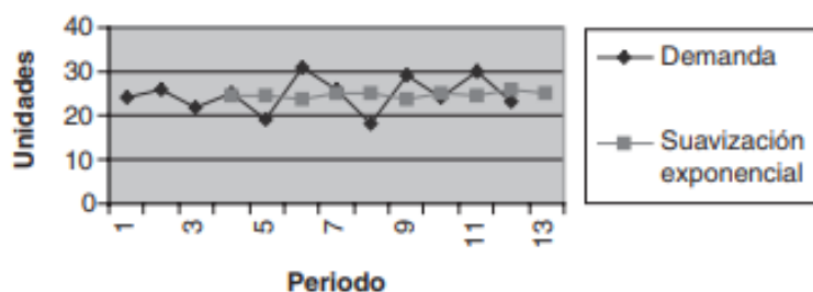
Figura 7. Suavización exponencial con \alpha = 0.2
