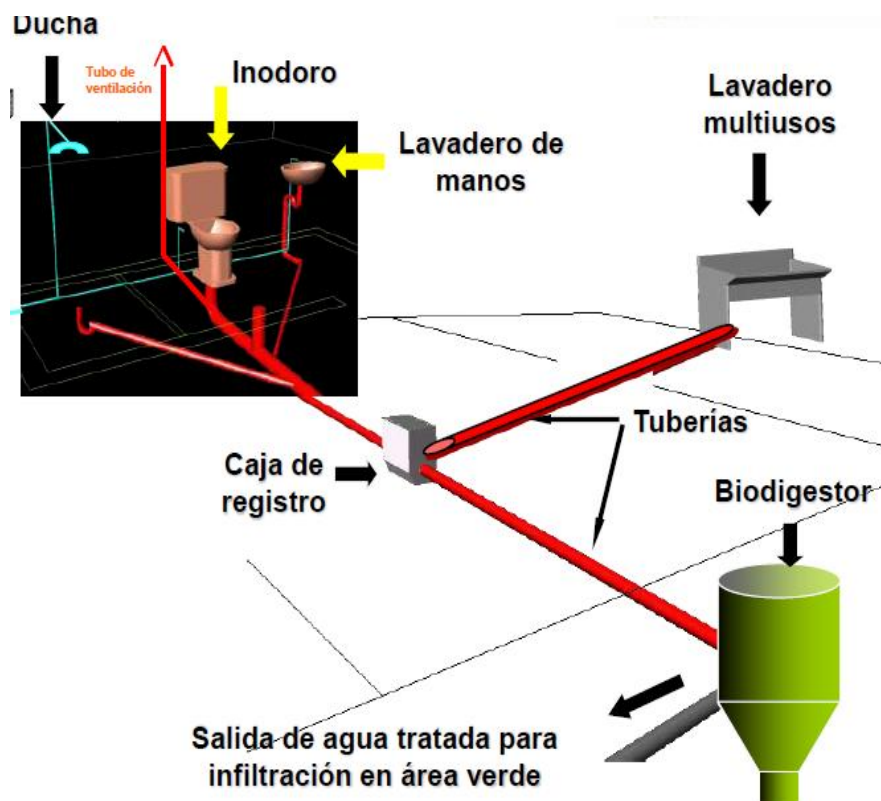
Figura 2. Unidad de Saneamiento Básico con Arrastre Hidráulico (UBS-AH)
