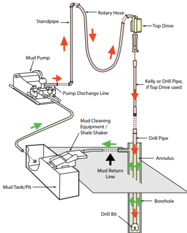
Рисунок 1.1 Базовая система циркуляции наземных буровых установок
