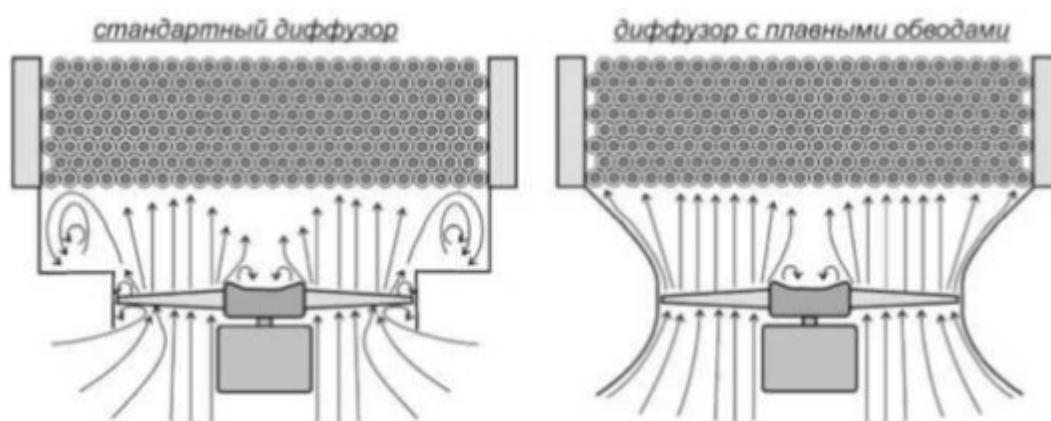
Рисунок 5 – Виды диффузора
