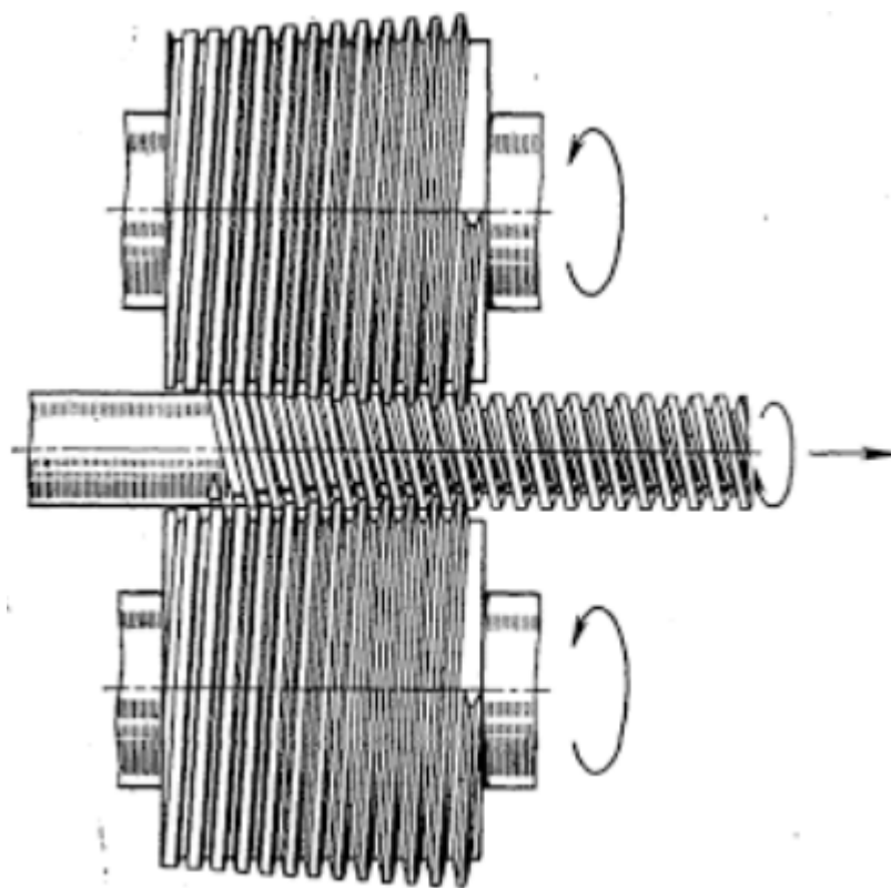
Рисунок 4 – Поперечно-винтовая прокатка
